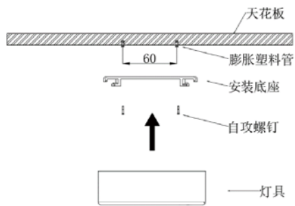
吸顶式照明灯安装示意图
