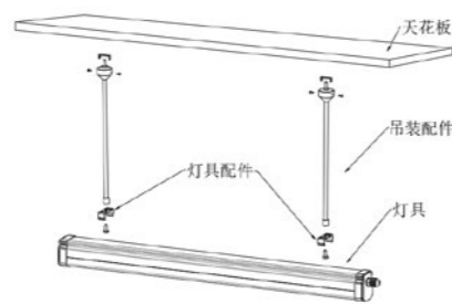
感应管灯安装示意图
