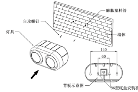
双头灯安装示意图
