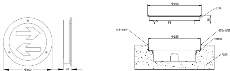
关键尺寸图 (mm)
