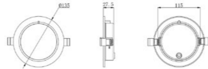
嵌顶式照明灯外形示意图(mm)
