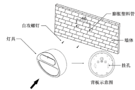
壁挂式照明灯安装示意图
