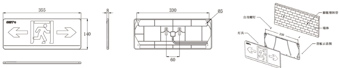
关键尺寸图 (mm)
